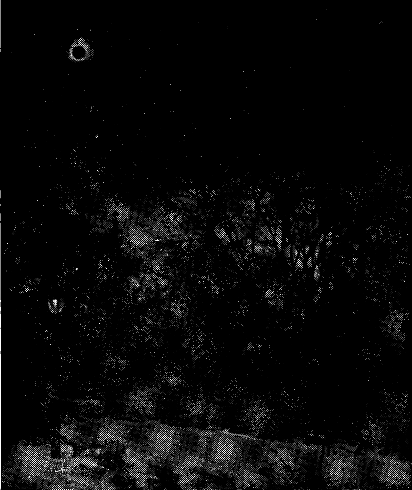
كسوف كامل در تمام اعصار باين شكل روى ميدهد شكل ۵- عكس كسوف كامل خورشيد در تاريخ ۲ ژانويه ۱۹۲۵ كه در برونكس پارک (Bronx park) نيويورك درفته شده .
