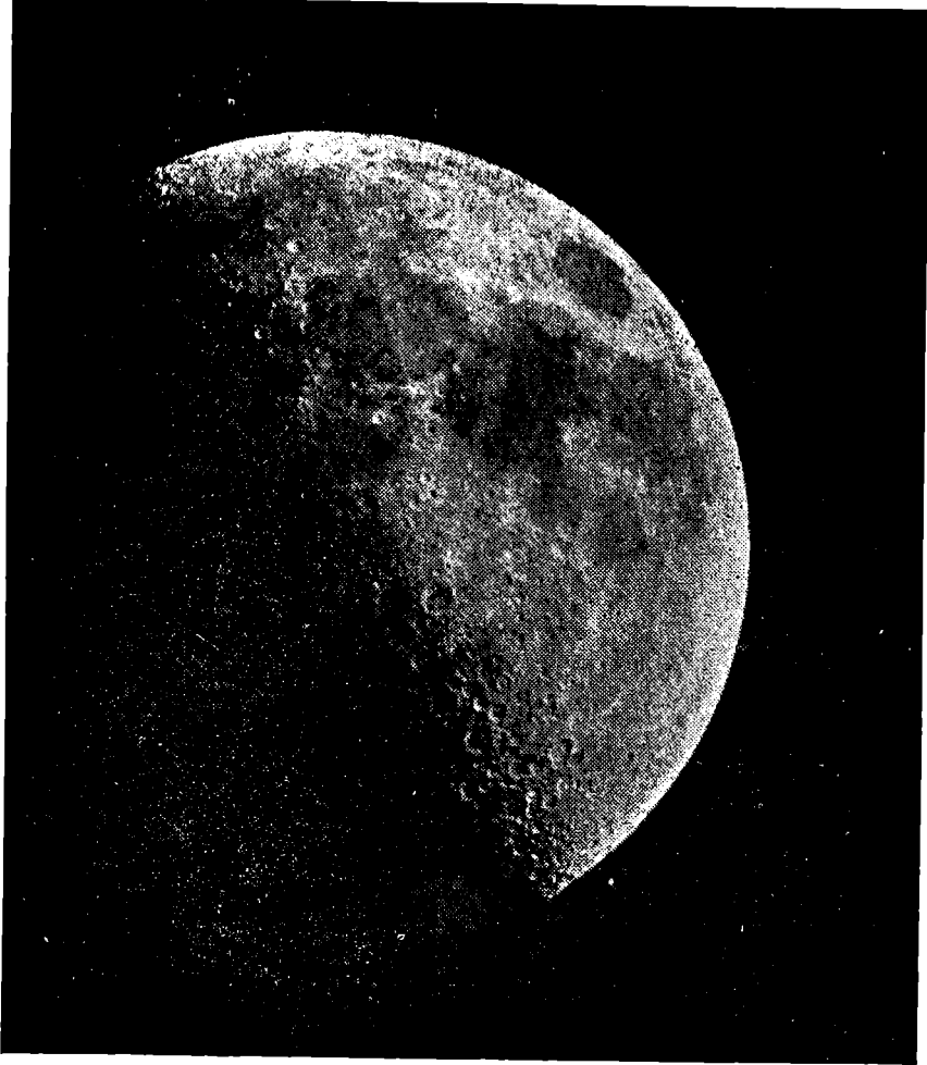
ماه شب هفتم شکل ۲۸ - (تربیع اول)
