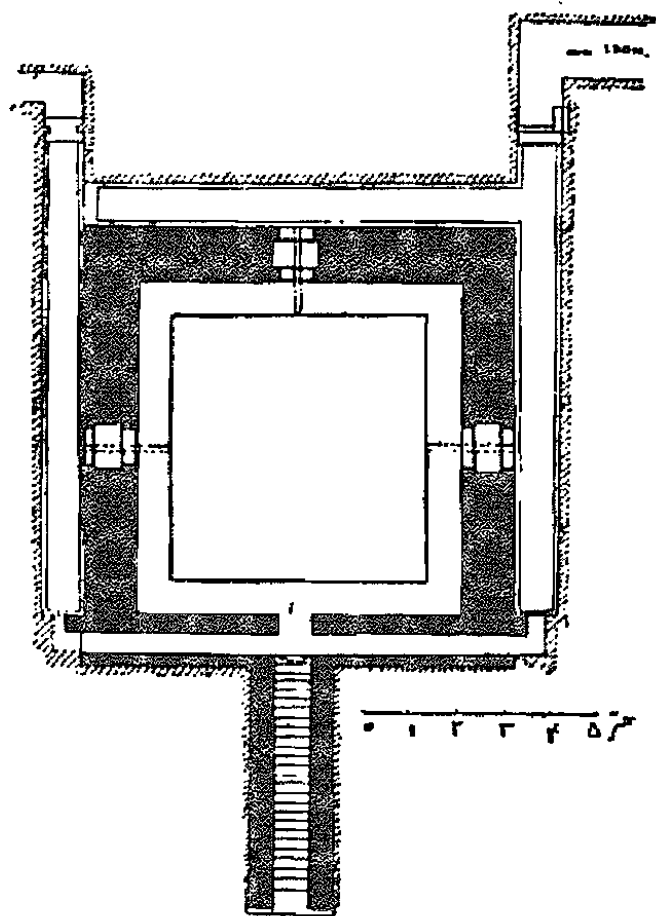
ش ۹۳- بیشاپور، نقشه آتشگاه
