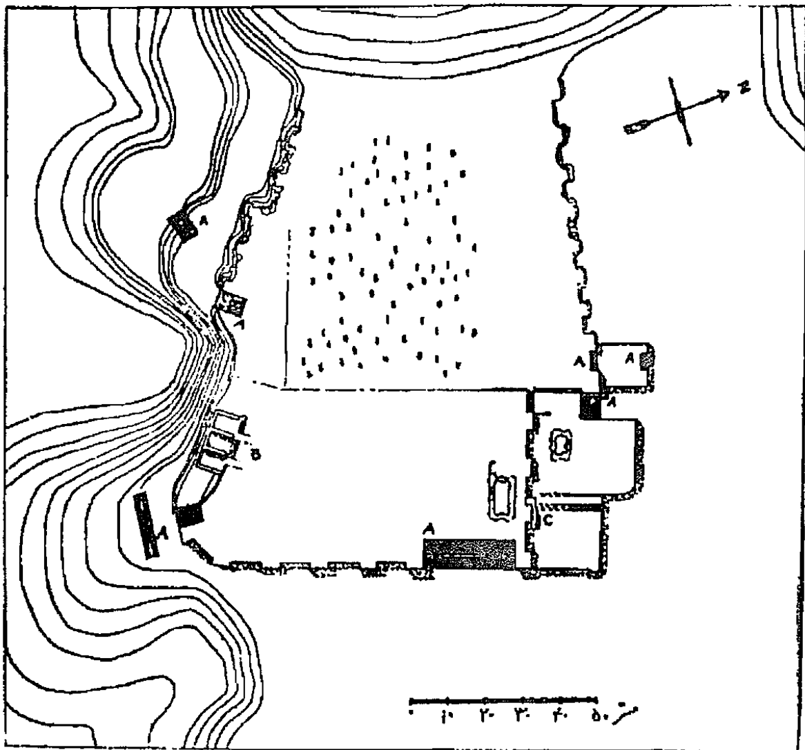
ش ۴۹- طرح تپه مسجد سلیمان
