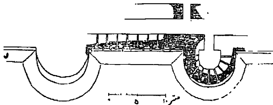
ش ۹۲ - استخر، دیوارگرد شهر، از خشت خام
