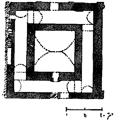
ش ۸۲ - هتره : طرح معبد
